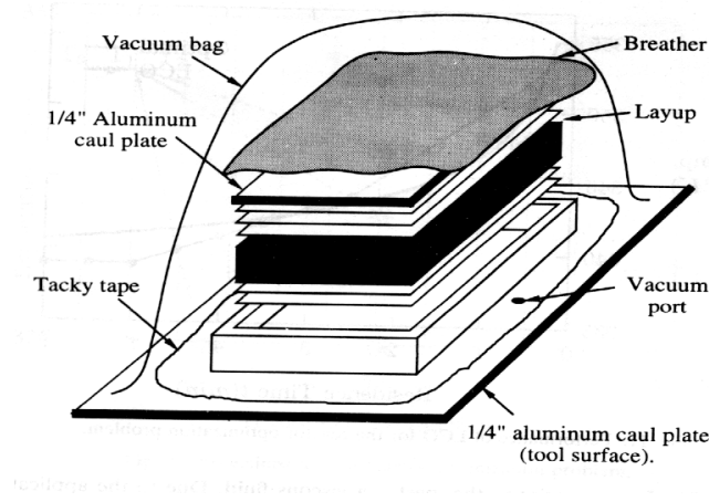
FIG. E.1 – Composite layup [10].
