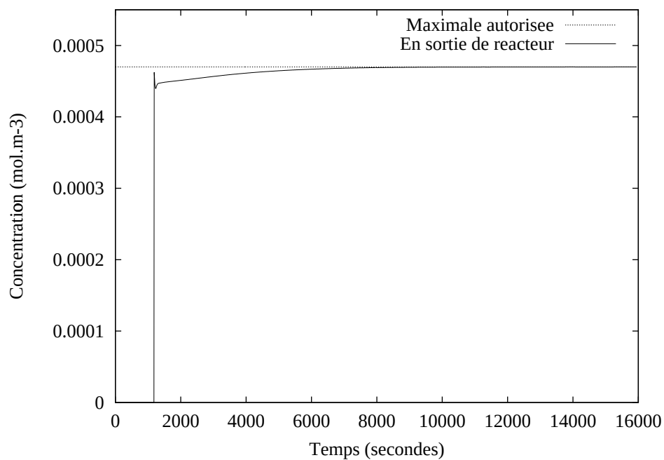
FIG. 6.16 – Concentration moyenne en sortie du procédé , (n_{mt}, n_{mc}, N_p) = (16, 16, 50s)
