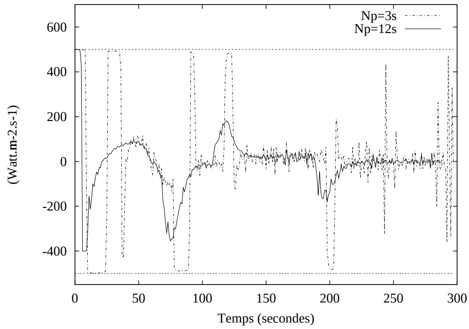
FIG. 7.14 – Vitesse de la commande pour N_p = 3s, 12s
