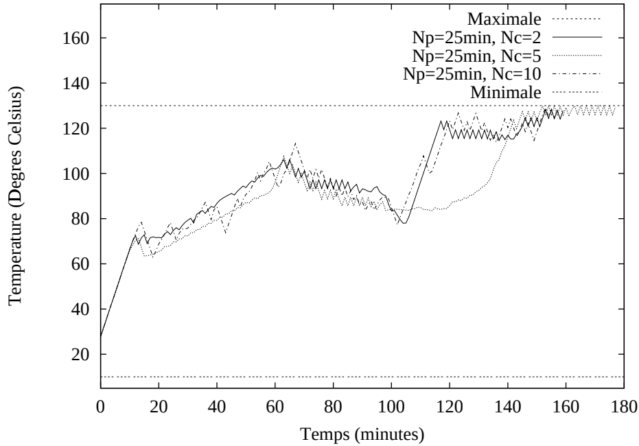
FIG. 5.13 – Température d'autoclave
