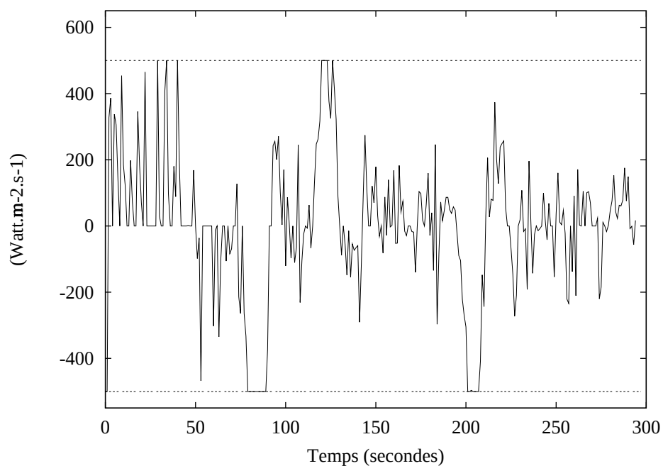
FIG. 7.21 – Vitesse de la commande pour N_p = 6s
