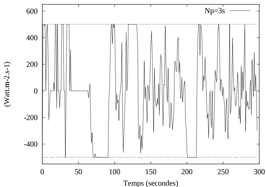
FIG. 7.20 – Vitesse de la commande pour N_p = 3s
