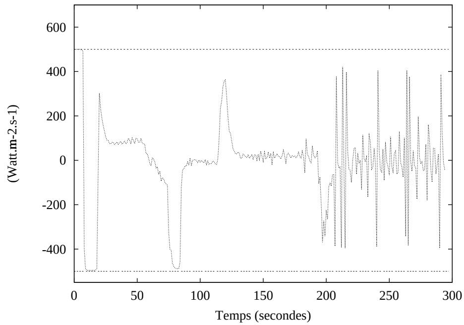
FIG. 7.15 – Vitesse de la commande pour N_p = 6s
