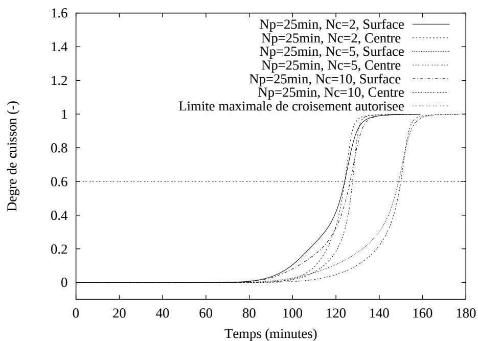
FIG. 5.21 – Degrés de cuisson dans le polymère
